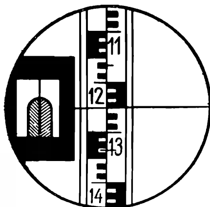
Рис. 73. Глухой нивелир НВ-1 (а) и поле зрения (б)
