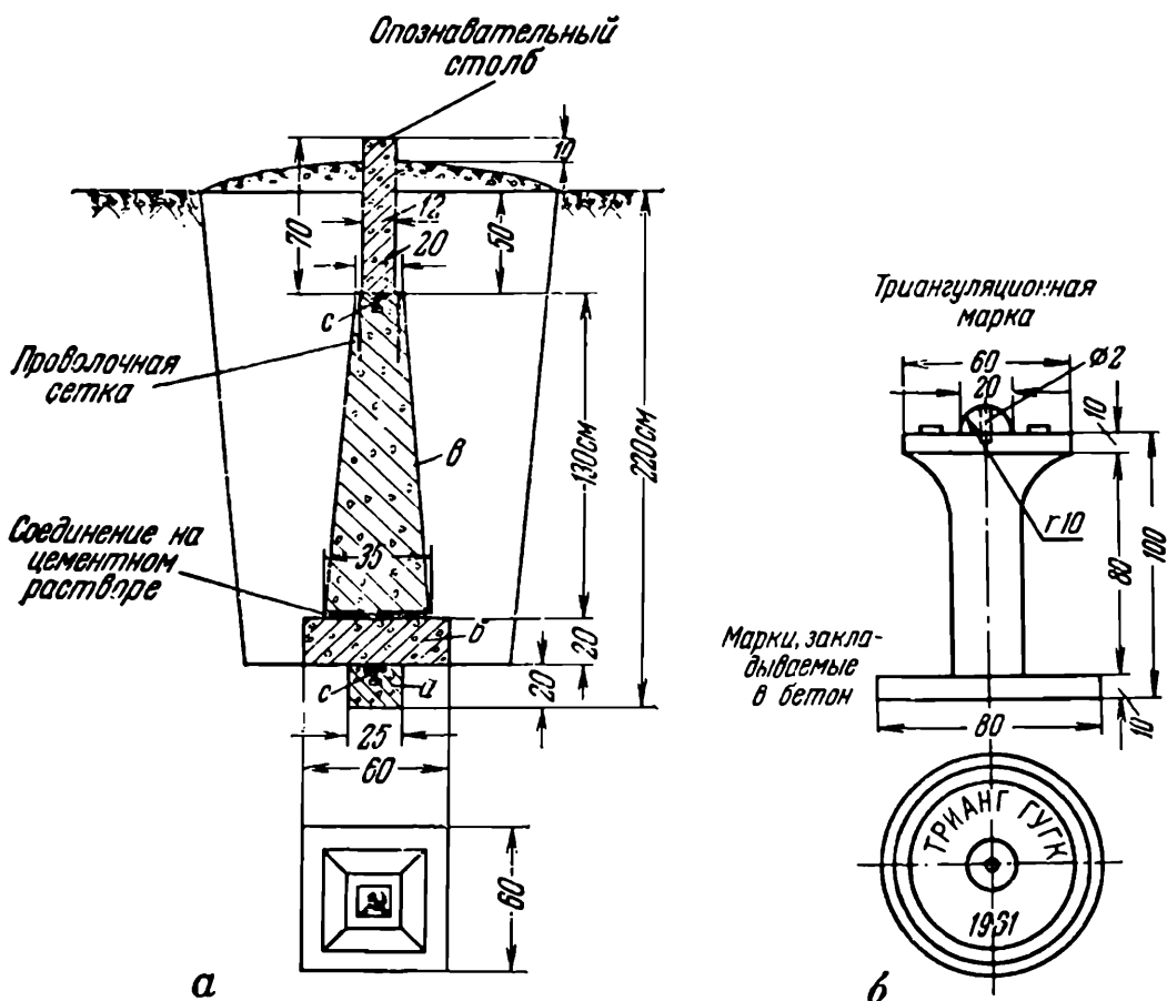
Рис. 38. Центр триангуляции 1, 2, 3, 4 классов
