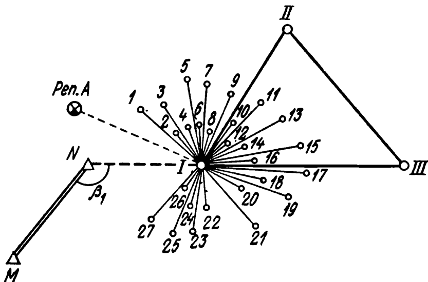
Рис. 99. Сомкнутый тахеометрический ход
