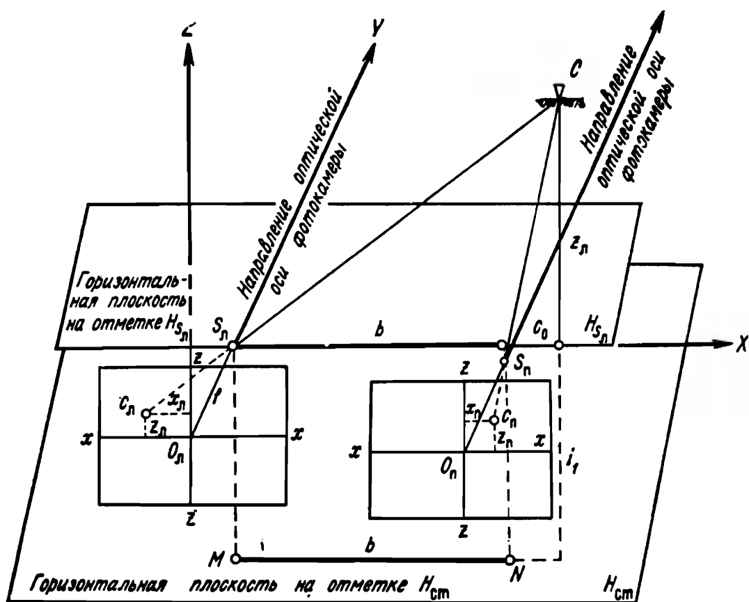
Рис. 107. Схема фотогеодезической съемки
