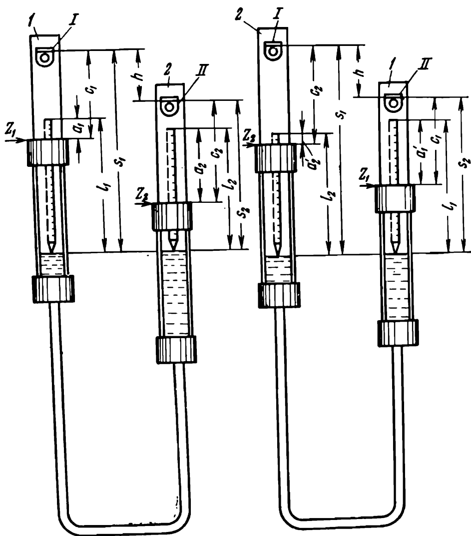
Рис. 116. Схема нивелирования прибором К. Терцаги
