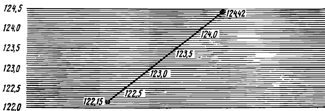
Рис. 89. Графическое интерполирование горизонталей
