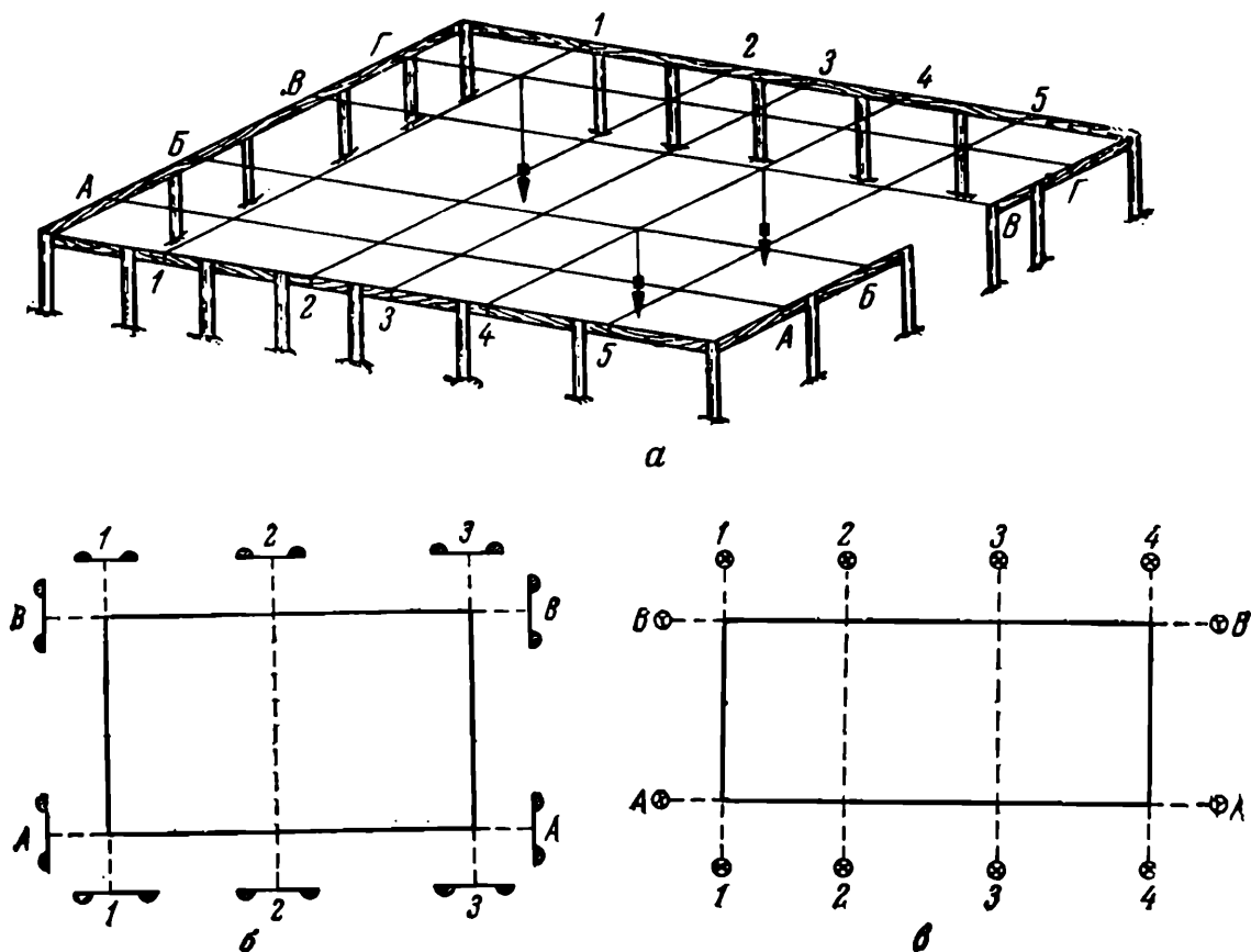
Рис. 145. Типы обноски
