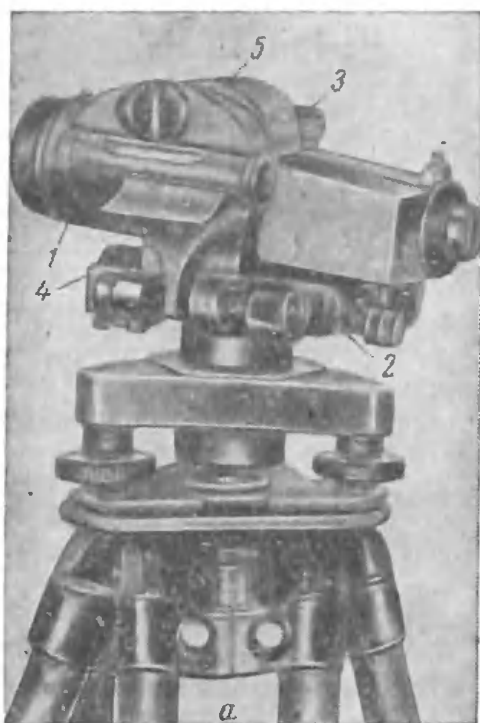
Рис. 75. Нивелир НЛ-3 (а) — оптический высотомер с прямолинейным высотным штрихом и поле зрения (б)
