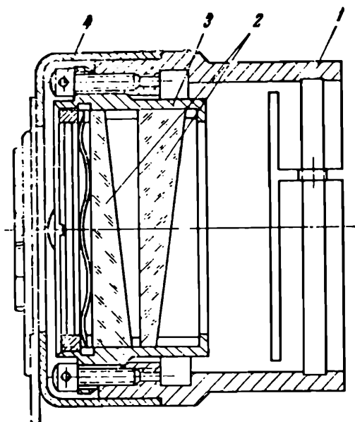
Рис. 9. Разрез насадки ДД-3
