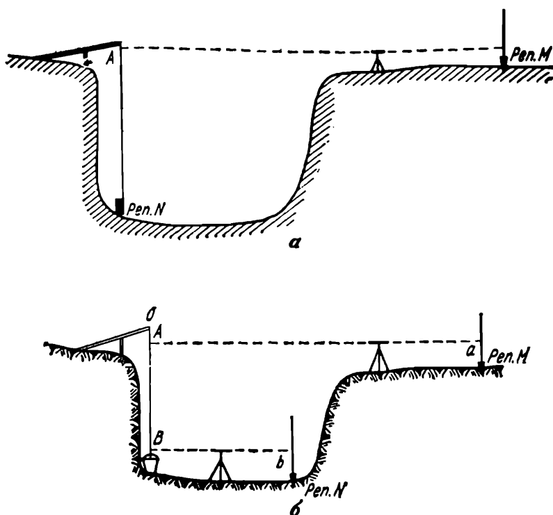
Рис. 139. Схема определения отметки точки в глубоком котловане
