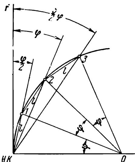
Рис. 166. Схема разбивки окружности при помощи эккера
