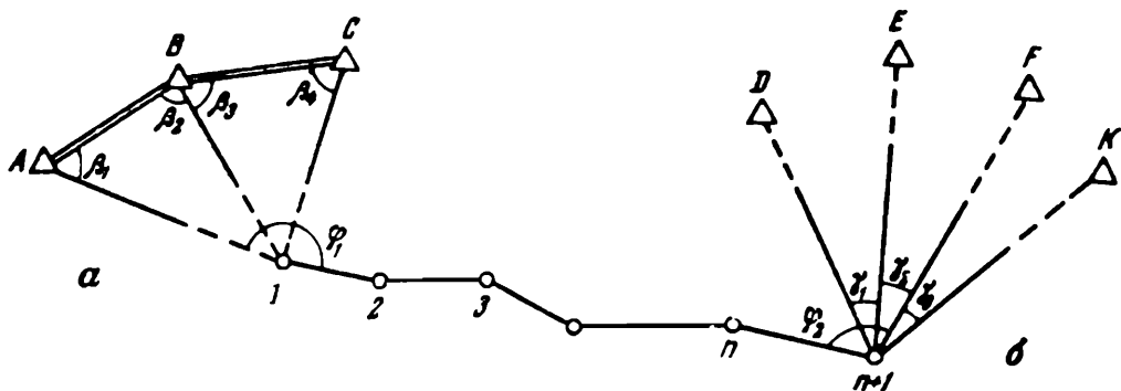
Рис. 45. Схема привязки теодолитного хода путем засечек
