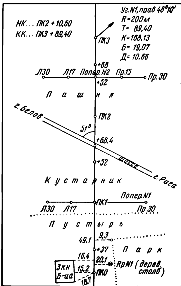
Рис. 80. Страница пикетажного журнала
