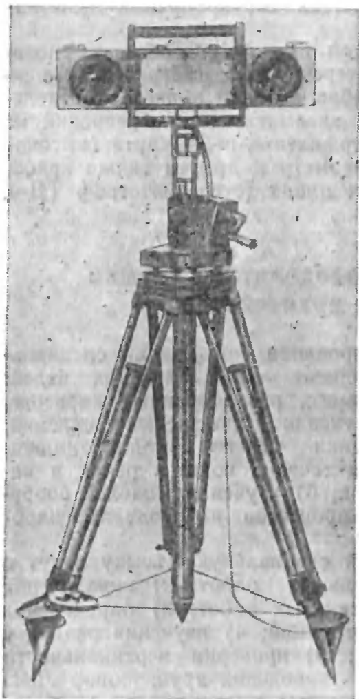
Рис. 110. Стереокамера
