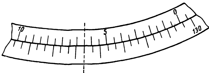
Рис. 16. Верньер 30-секундного теодолита
