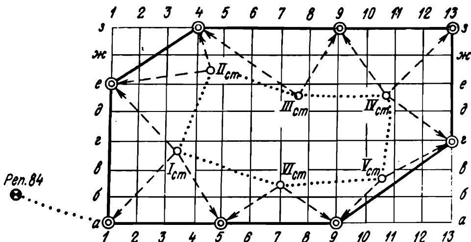
Рис. 87. Схема нивелирования связующих точек
