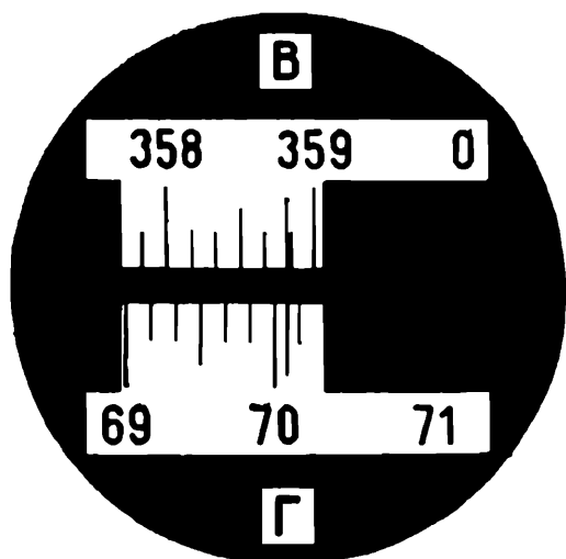
Рис. 21. Поле зрения отсчетного микроскопа теодолита Т30
