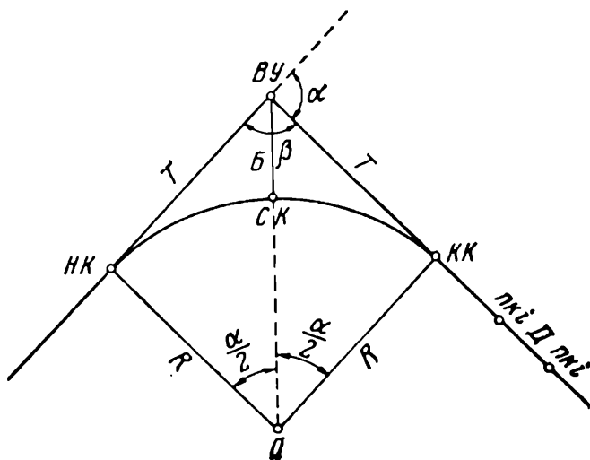
Рис. 81. Схема разбивки кривой тремя главными точками
