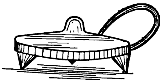
Рис. 79. Башмак для установки нивелирной рейки
