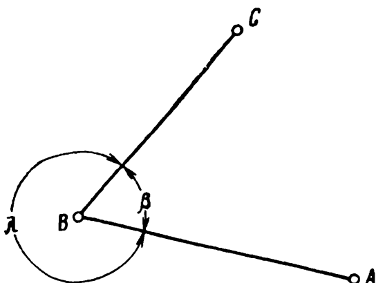
Рис. 25. Измеряемые горизонтальные углы \beta и \lambda
