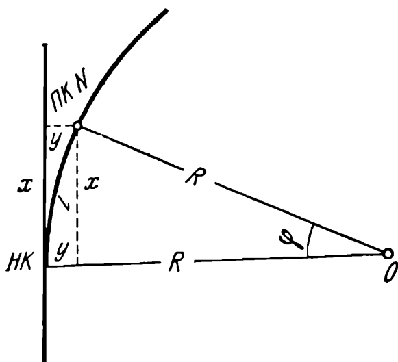
Рис. 82. Схема выноса пикета на кривую
