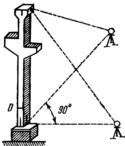
Рис. 151. Проверка установки колонны
