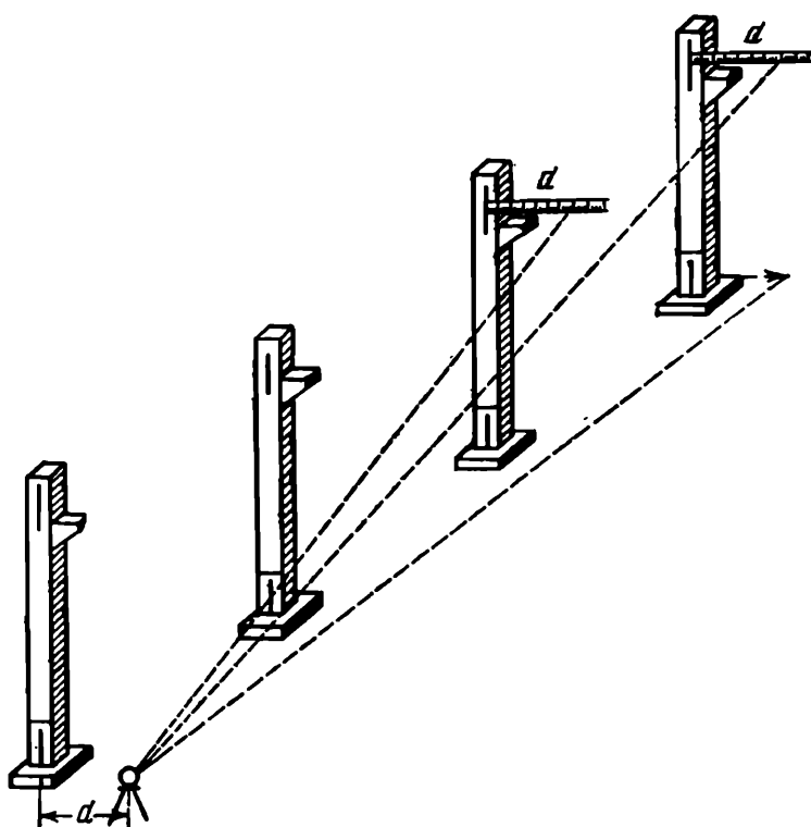
Рис. 152. Проверка установки ряда колонн
