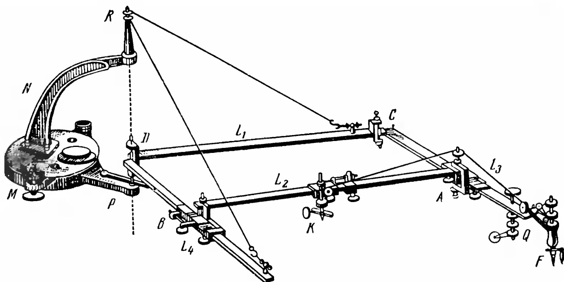
Рис. 65. Пантограф
