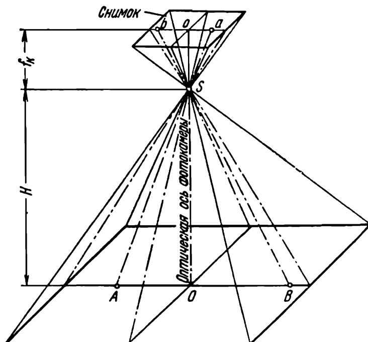
Рис. 111. Схема фотографирования с самолета
