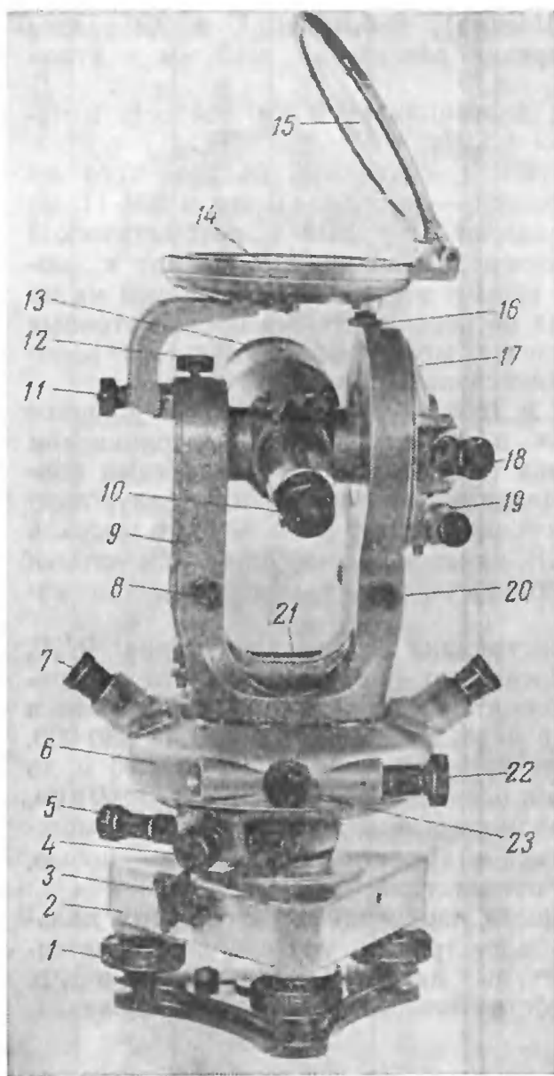
Рис. 12. Теодолит-тахеометр ТТ-5
