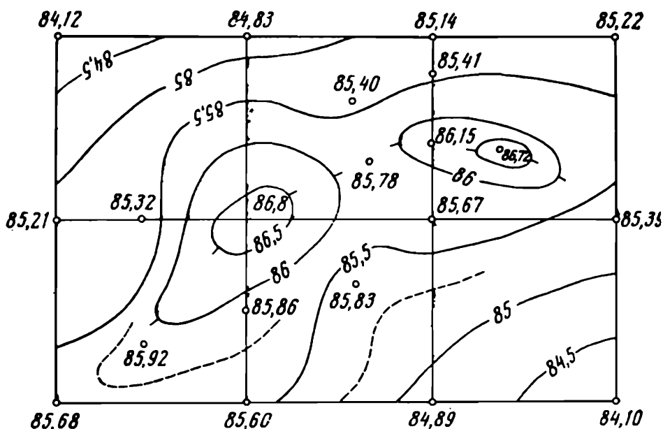
Рис. 90. Рельеф, изображенный горизонталями по отметкам точек квадратов
