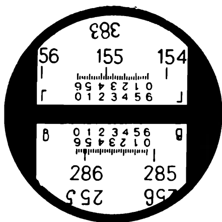
Рис. 22. Поле зрения отсчетного микроскопа теодолита Т20
