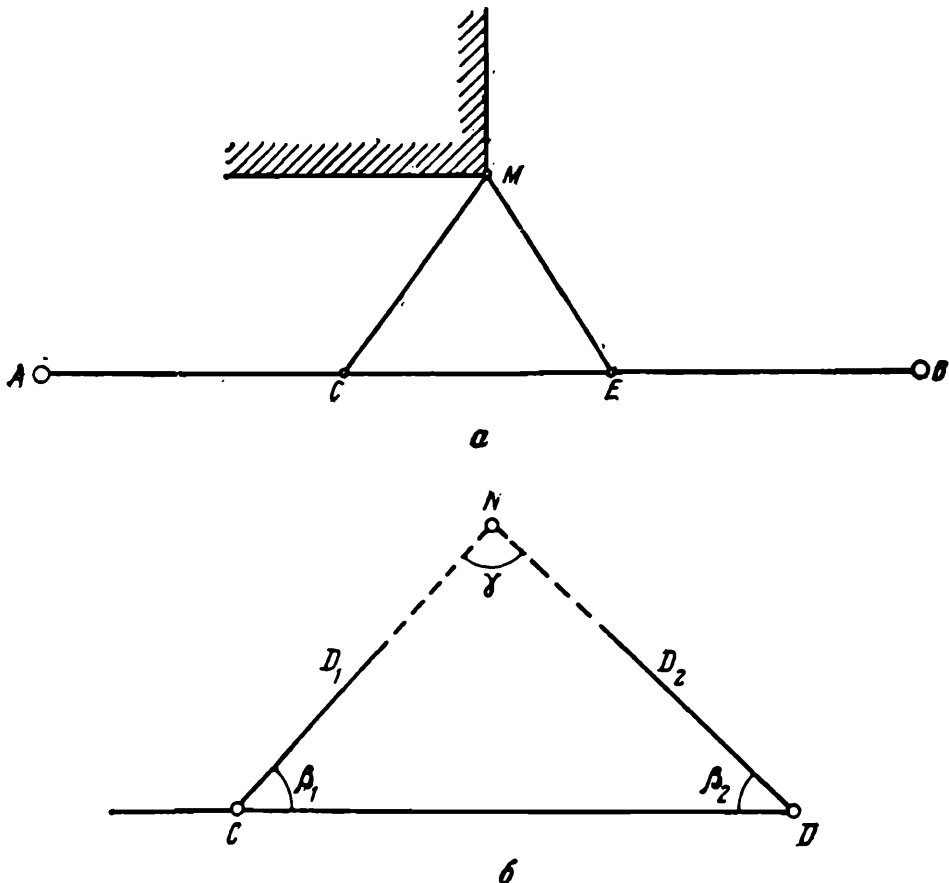
Рис. 53. Съемка способом засечек а — линейная; б — угловая
