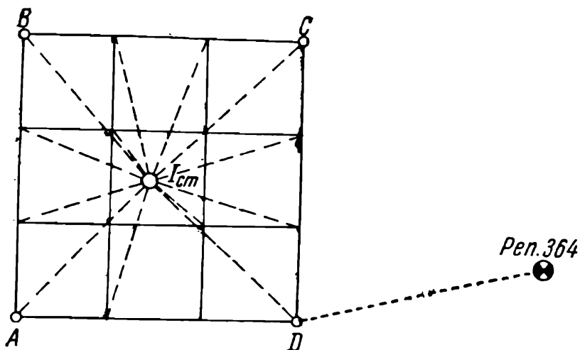
Рис. 86. Схема нивелирования участка с одной станции
