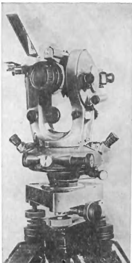
Рис. 14 Теодолит ТН
