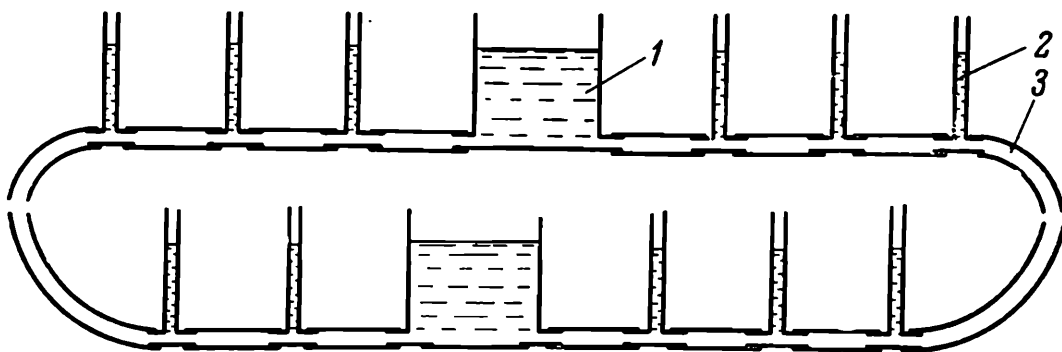
Рис. 117. Гидростатическая система
