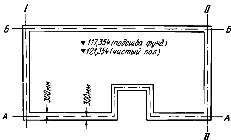
Рис. 174. Разбивочный чертеж фундамента наружных стен
