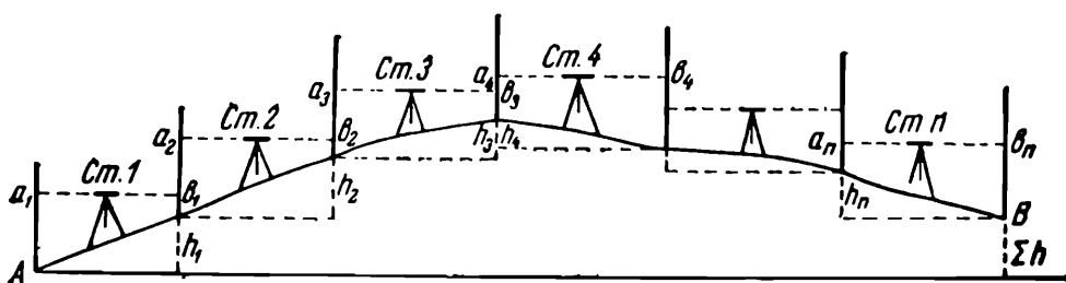
Рис. 68. Нивелирный ход
