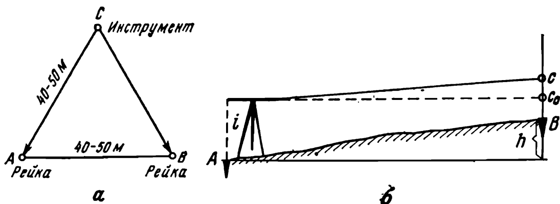
Рис. 70. Проверка главного условия глухого нивелира первым способом
