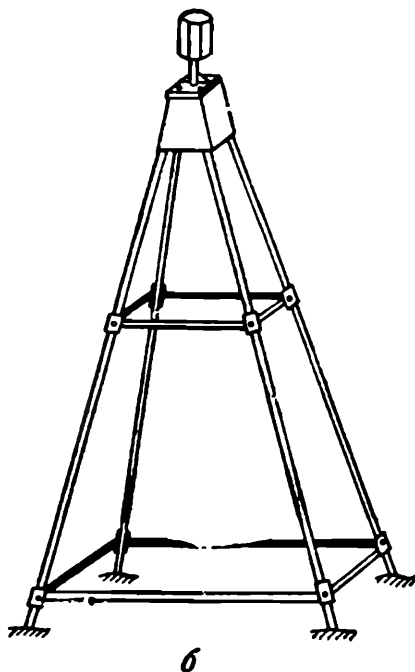
Рис. 39. Наземные сооружения на пунктах триангуляции
