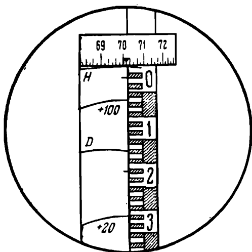
Рис. 97. Поле зрения зрительной трубы тахеометра ТА-2
