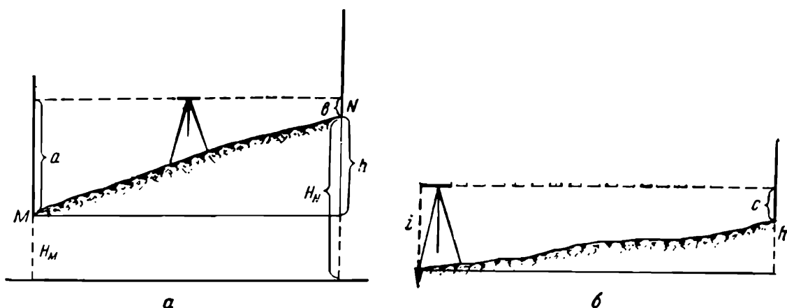
Рис. 67. Два способа геометрического нивелирования
