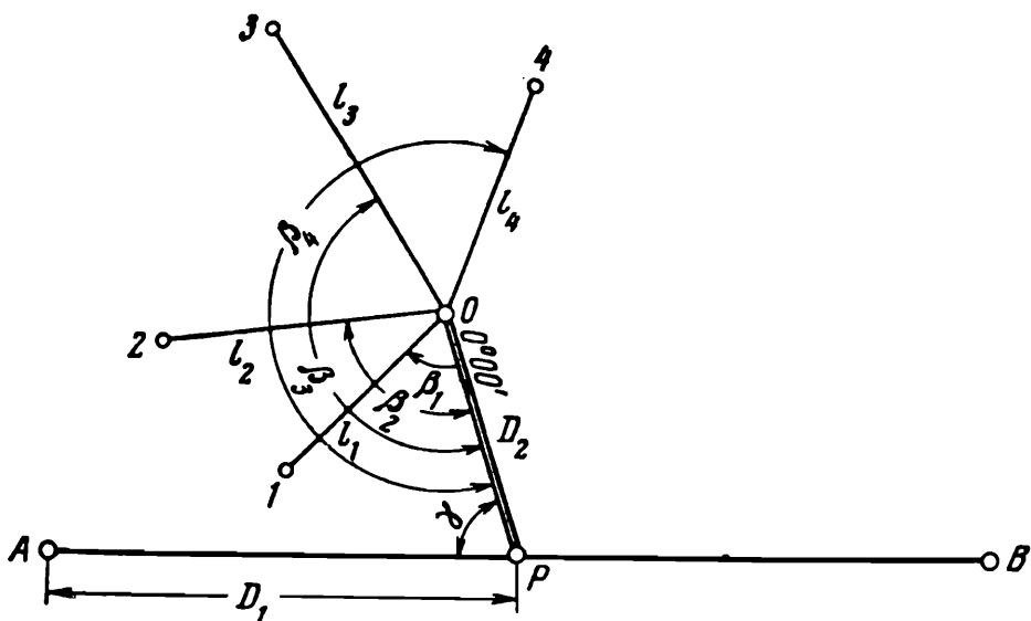
Рис. 54. Съемка полярным способом
