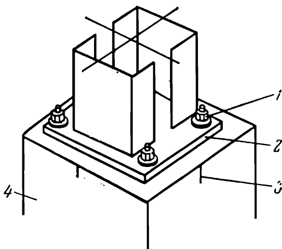
Рис. 147. Нижняя часть стальной колонны 1 — анкерные болты; 2 — башмак; 3 — осевые риски; 4 — фундамент
