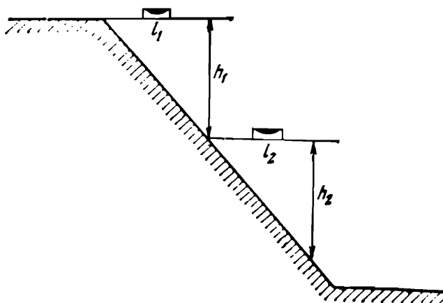
Рис. 93. Ватерпасовка кру- тых склонов
