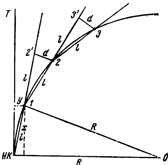
Рис. 164. Схема разбивки кривой по способу продолженных хорд
