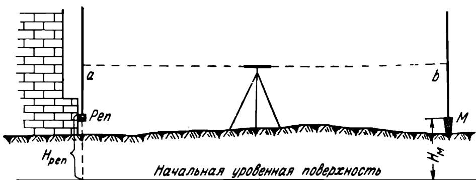
Рис. 134. Репер и искомая точка ниже горизонта инструмента
