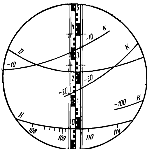
Рис. 102. Поле зрения трубы кипрегеля КБ-1
