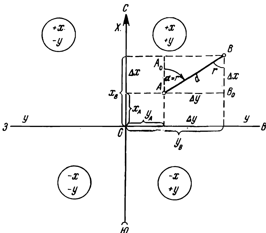
Рис. 36. Система плоских прямоугольных координат, применяемая в геодезии
