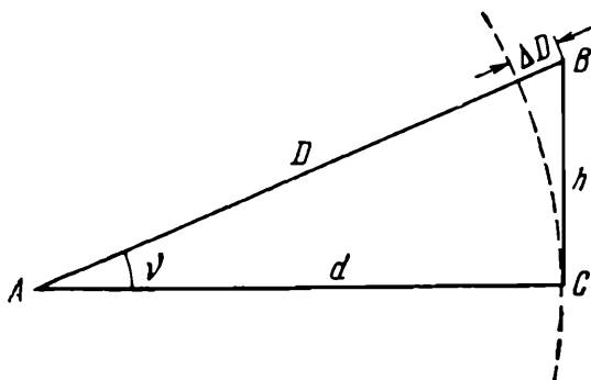
Рис. 2. Поправка за наклон линии к горизонту
