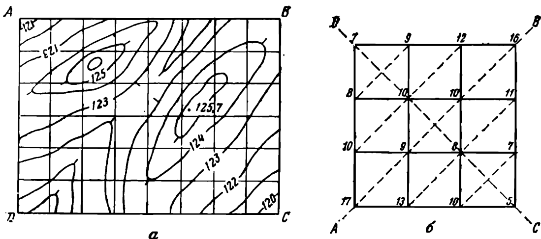
Рис. 128. Сетка квадратов, построенная на топографической карте
