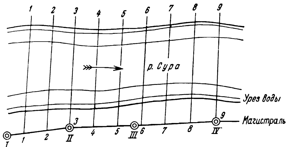
Рис. 92. Схема съемки водоемов на основе теодолитно-нивелирной магистрали с поперечниками
