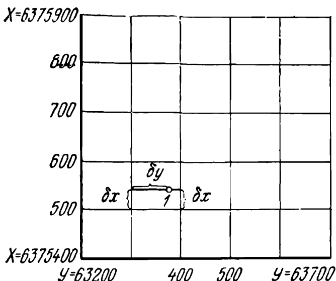
Рис. 60. Подпись координатной сетки и нанесение точек по координатам
