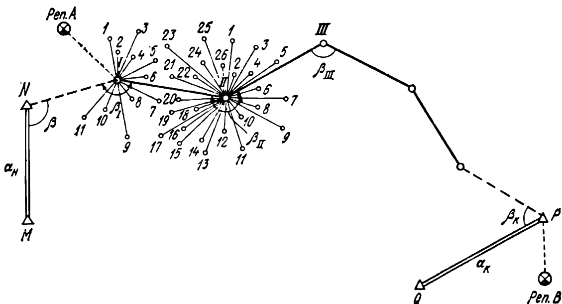
Рис. 98. Разомкнутый тахеометрический ход
