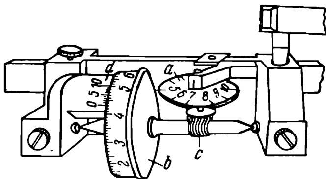
Рис. 64. Счетный механизм планиметра
