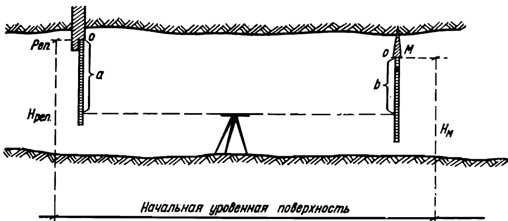
Рис. 136. Репер и искомая точка выше горизонта инструмента
