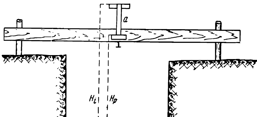
Рис. 154. Обноска на траншее с постоянной визиркой
