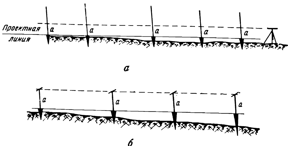
Рис. 157. Схема разбивки наклонной проектной линии при помощи наклонного луча визирования в нивелир и по визиркам
