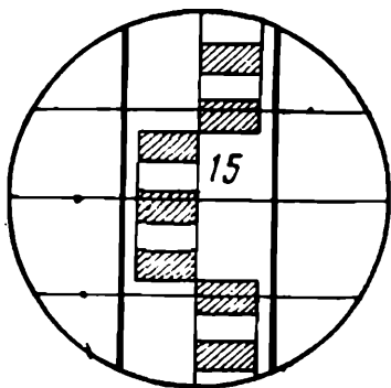
Рис. 78. Отсчет по рейке
