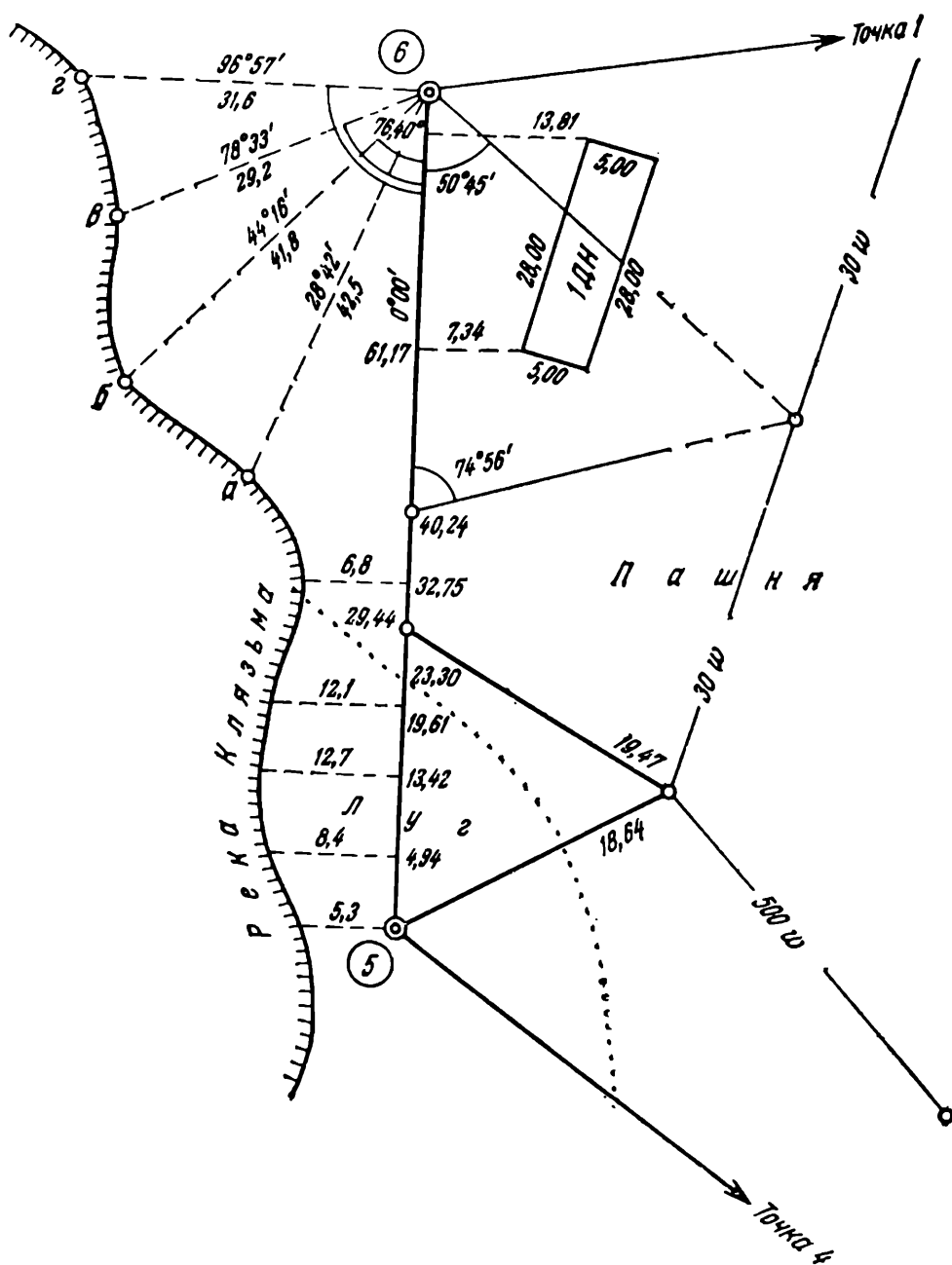
Рис. 58. Абрис съемки
