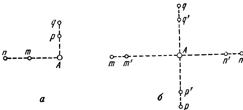
Рис. 144. Схема закрепления точки A створами mn и pq
