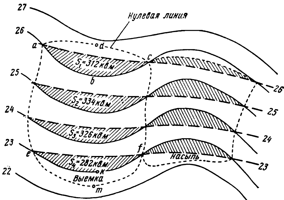
Рис. 131. Определение объемов насыпи и выемки по горизонталям
