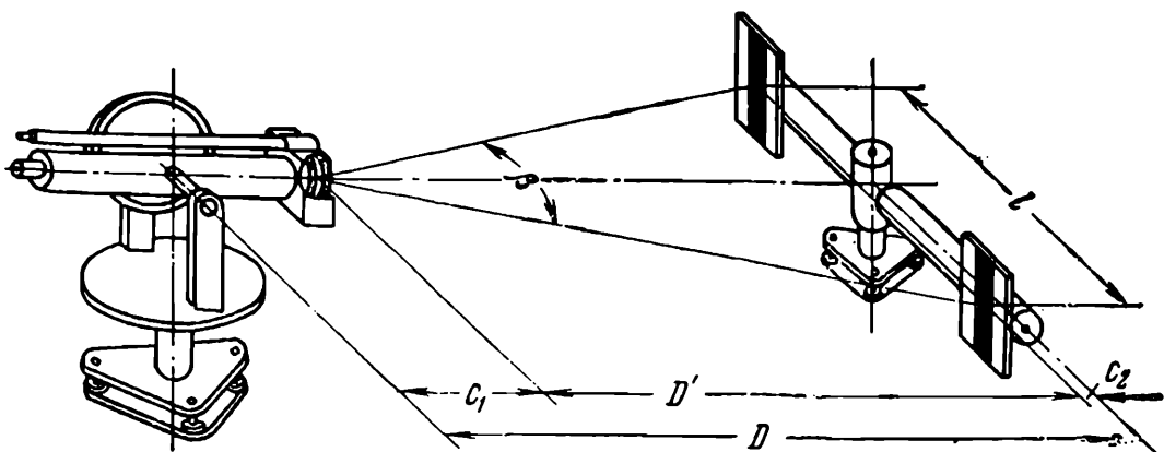
Рис. 4. Схема действия дальномера ДНТ
