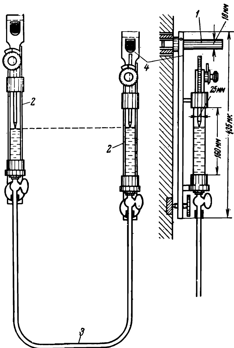
Рис. 115. Гидростатический прибор К. Терцаги
