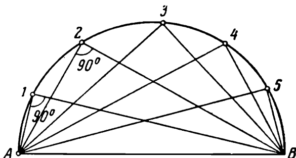
Рис. 166. Схема разбивки окружности при помощи эккера
