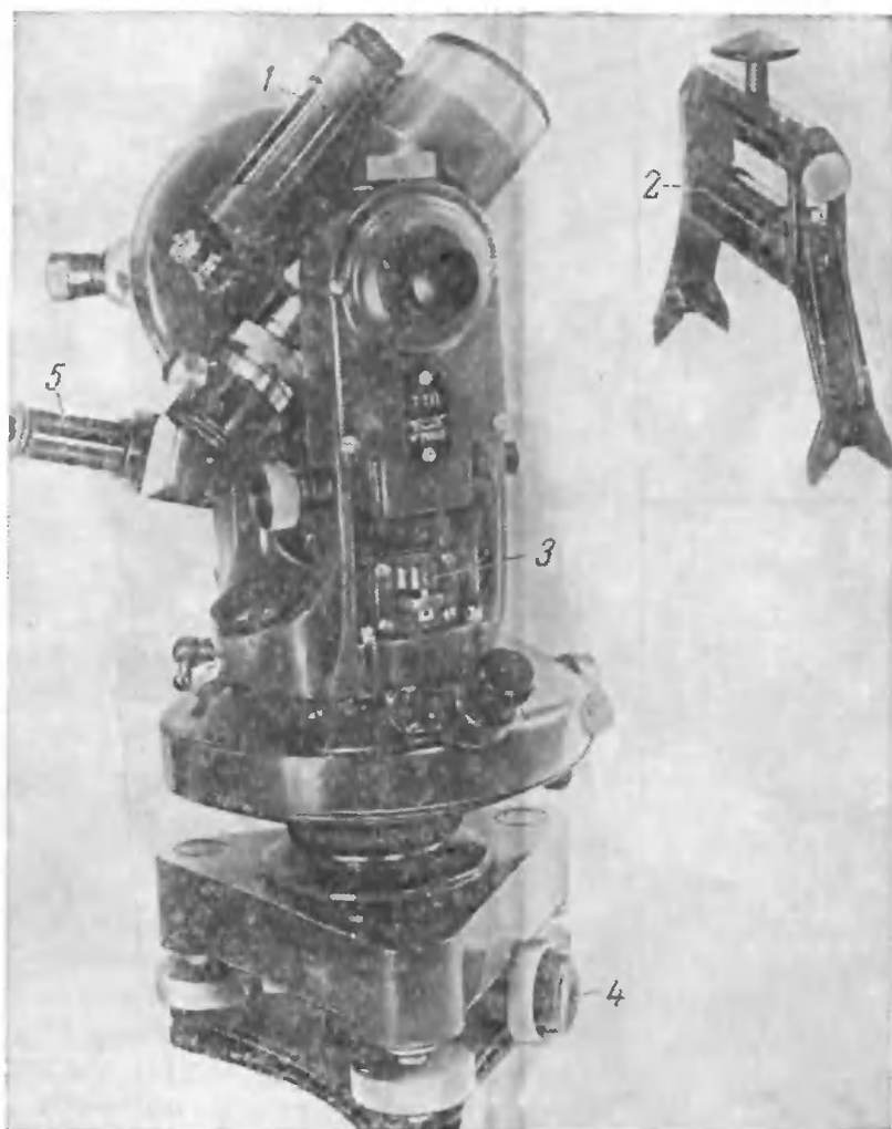
Рис. 13. Теодолит ТТП
