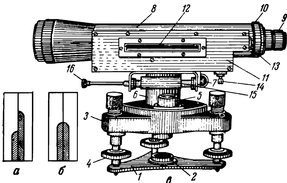
Рис. 69. Глухой нивелир (НГ) с контактным уровнем
