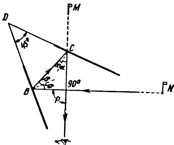
Рис. 52. Схема построения прямого угла экером
