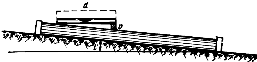
Рис. 155. Схема укладки труб по уровню
