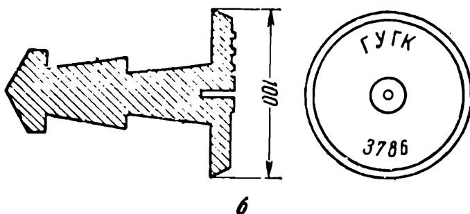
Рис. 41. Типы стенных нивелирных знаков
