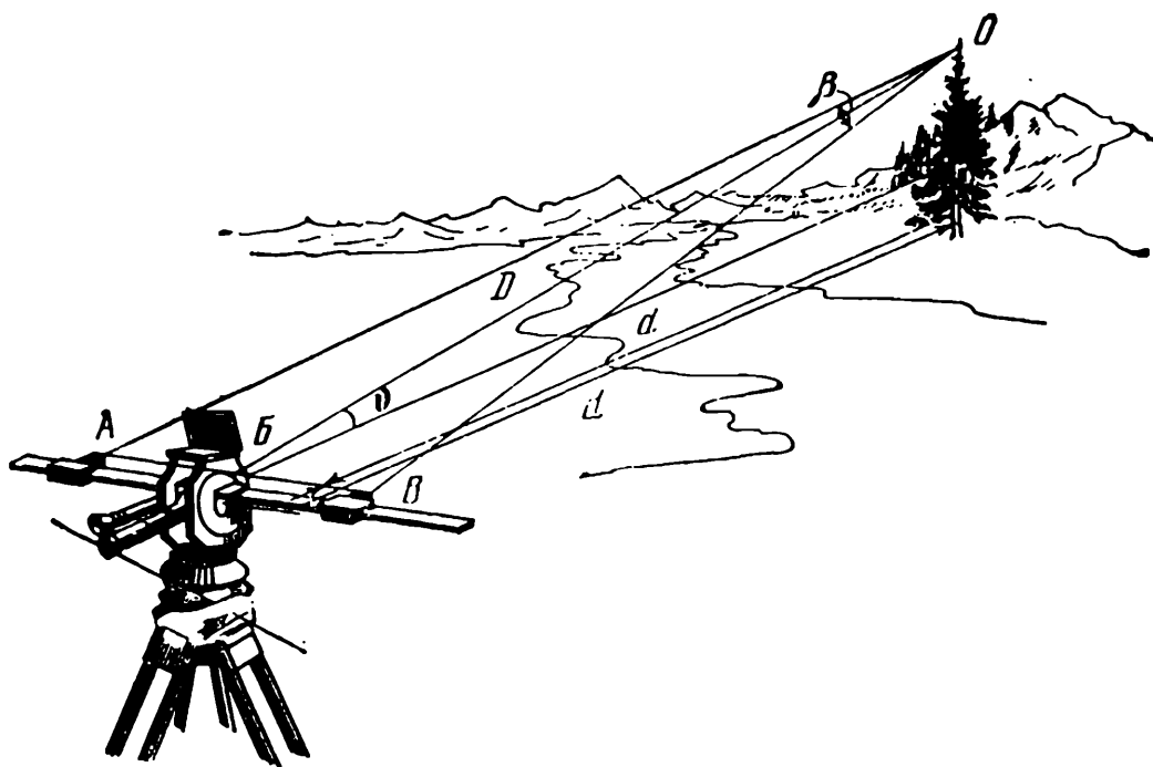
Рис. 11. Схема измерения расстояний дальномером ДВГ
