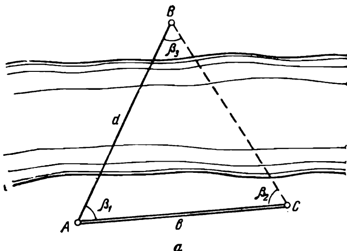
Рис. 48. Схема определения расстояния, недоступного для непосредственных измерений
