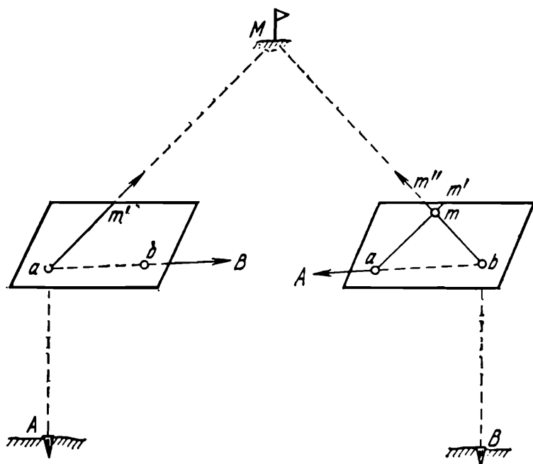
Рис. 104. Прямая мензульная засечка
