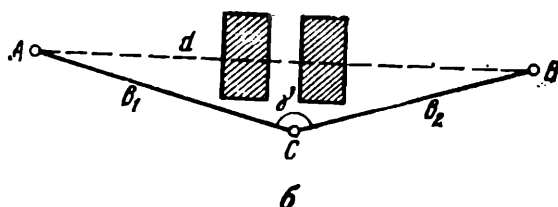
Рис. 48. Схема определения расстояния, недоступного для непосредственных измерений
