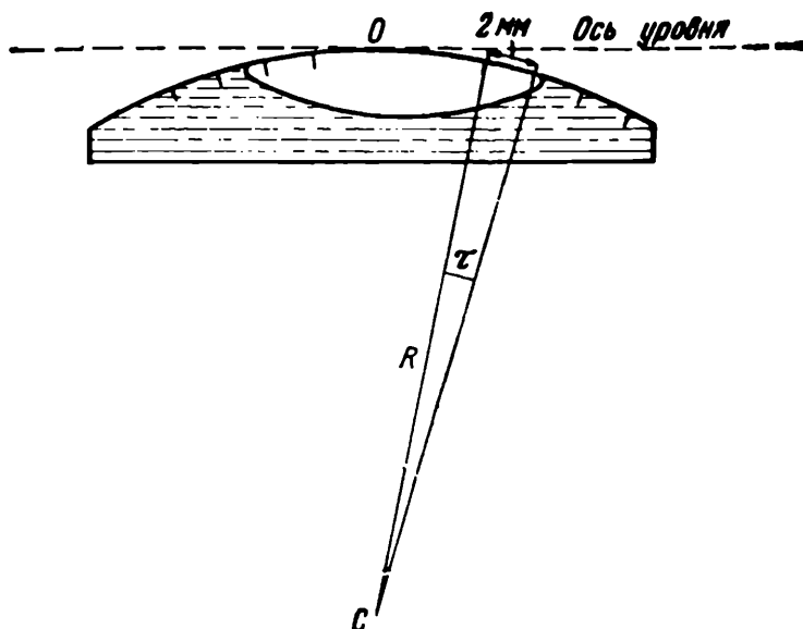
Рис. 17. Цилиндрический уровень
