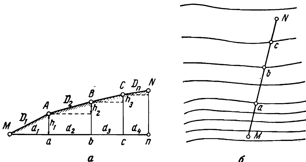
Рис. 126. Схема определения по карте длины наклонных линий
