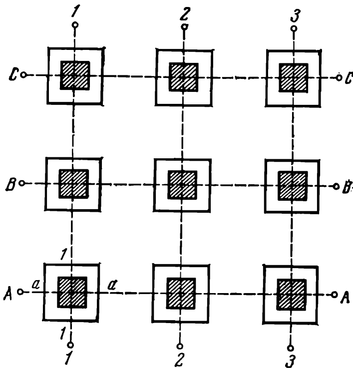
Рис. 149. Обозначение осей колонн на фундаментах
