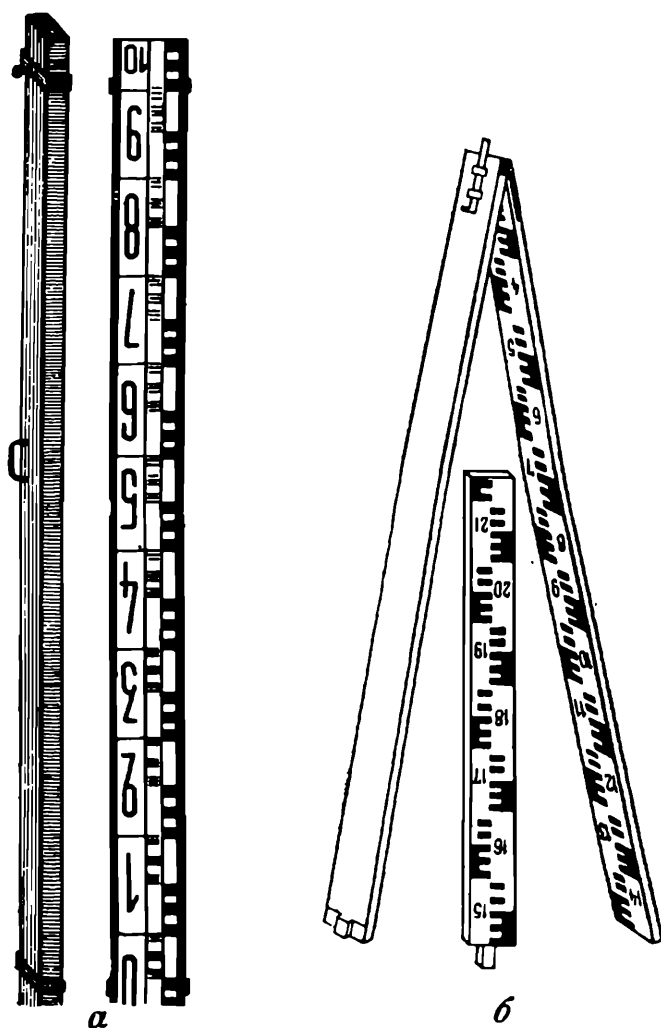
Рис. 77. Нивелирные рейки
