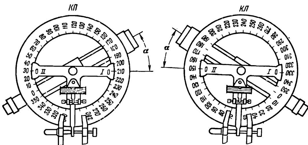
Рис. 28. Вертикальный круг тахеометра
