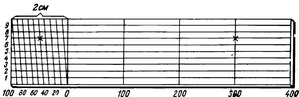
Рис. 58. Поперечный масштаб для вычисленного масштаба 1 : 5000
