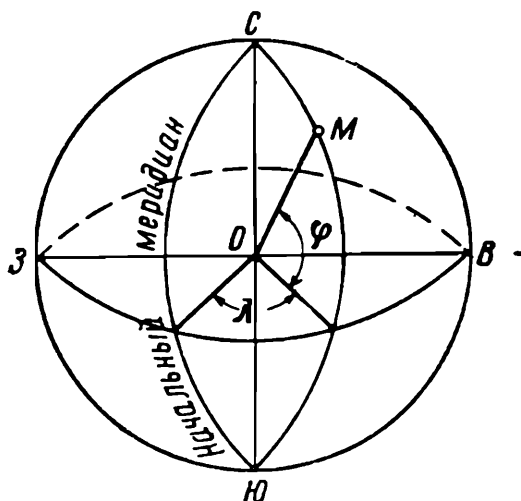
Рис. 34. Географические координаты в изображении на шаре
