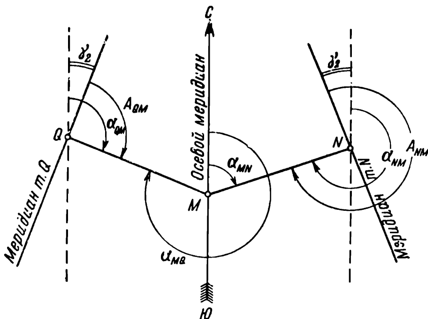
Рис. 30. Сближение меридианов в зоне системы координат Гаусса
