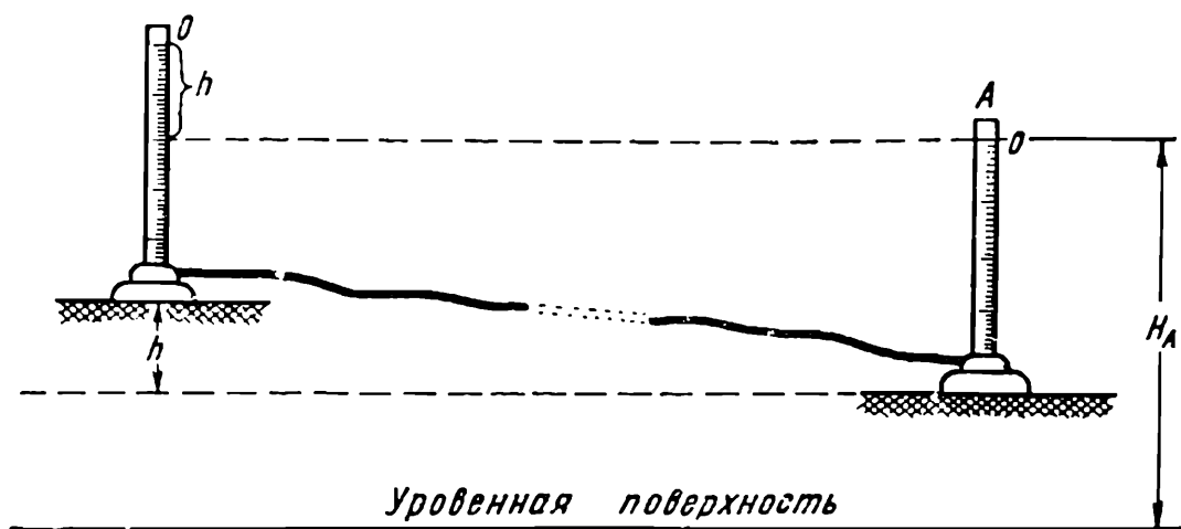
Рис. 114. Гидростатическое нивелирование
