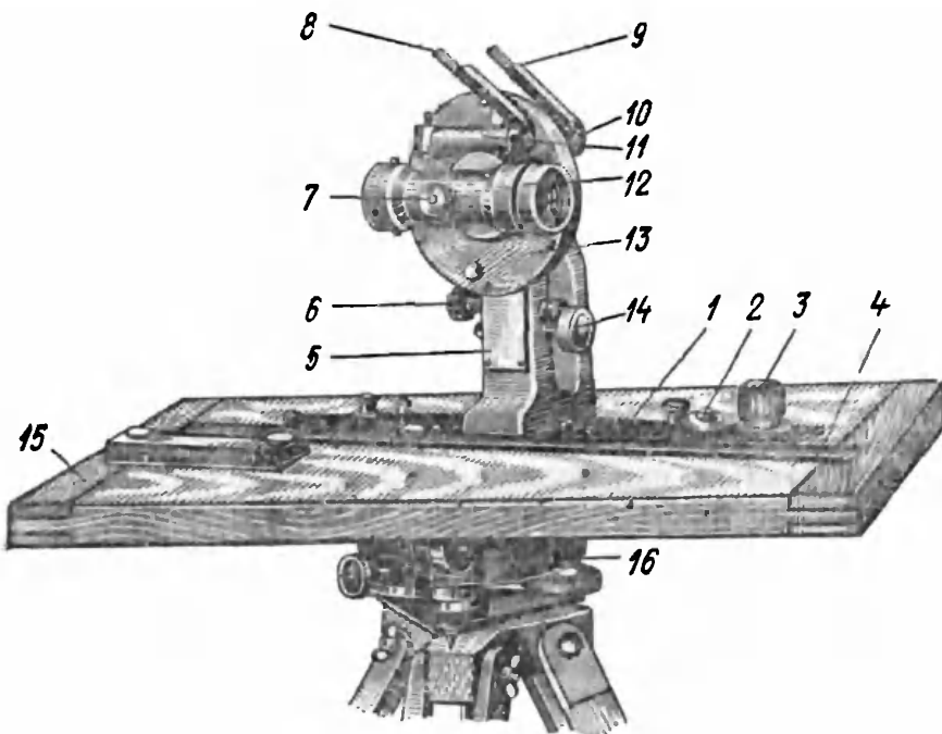
Рис. 101. Мензула и кипрегель КБ-1
