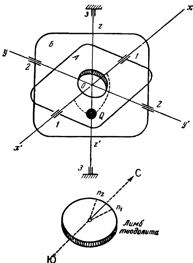
Рис. 33. Схематическое изображение маятникового гироскопа
