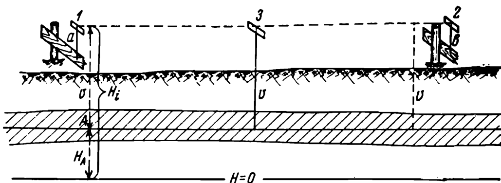
Рис. 153. Постоянная и ходовые визирки
