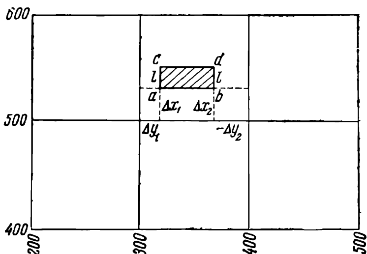
Рис. 141. Схема привязки здания к строительной сетке
