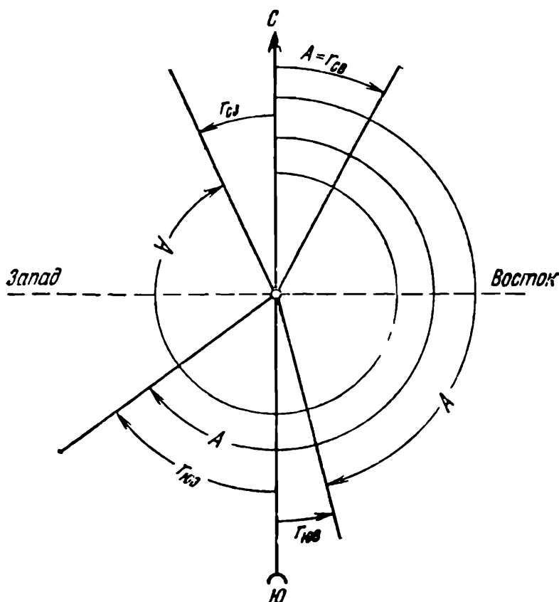
Рис. 28. Азимуты и румбы линий
