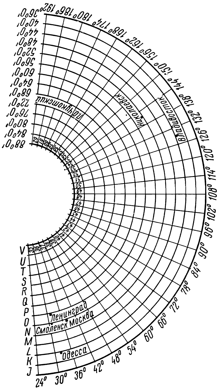
Рис. 119. Разграфка и номенклатура листов карты масштаба 1 : 1 000 000
