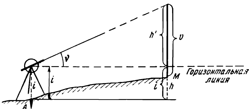
Рис. 95. Определение высотного положения точки M
