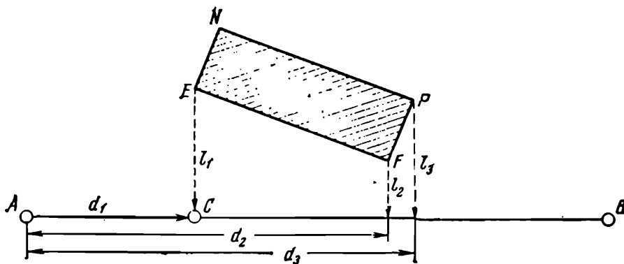
Рис. 49. Съёмка здания по способу перпендикуляров
