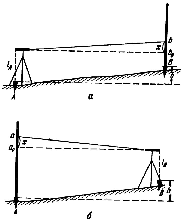
Рис. 71. Проверка главного условия глухого нивелира вторым способом
