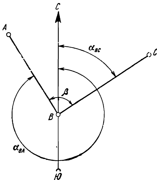
Рис. 124. Изображение горизонтального угла, равного разности дирекционных углов
