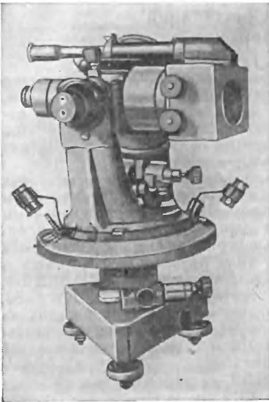
Рис. 5. Дальномерная насадка ДНТ на трубе теодолита
