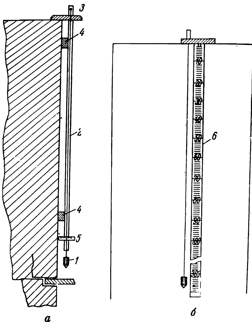
Рис. 146. Отвес-линейка
