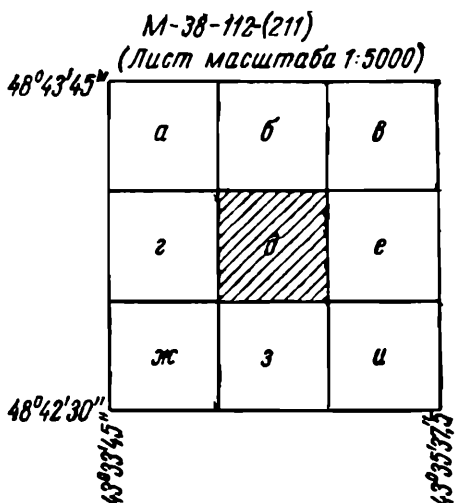
Рис. 120. Разграфка и номенклатура топографических карт
