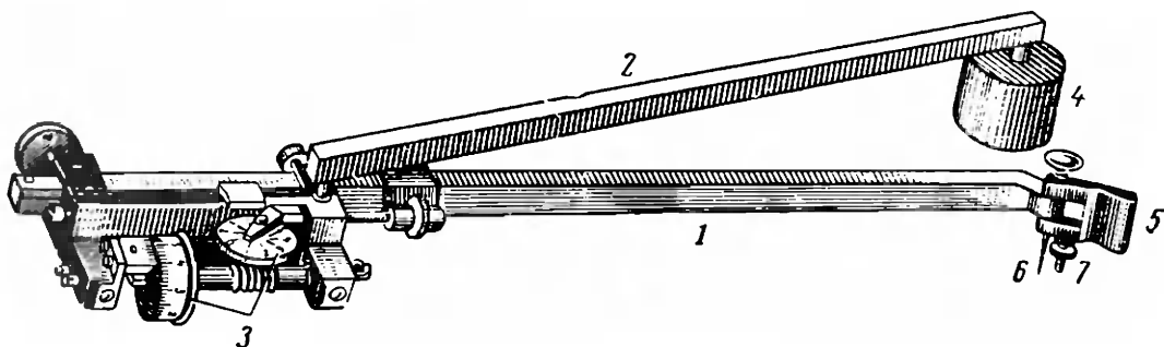
Рис. 62. Полярный планиметр
