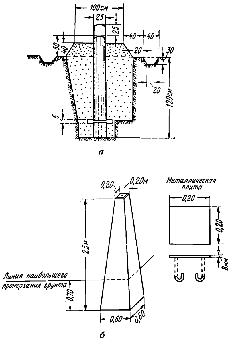
Рис. 43. Типы знаков для закрепления точек строительной сетки
