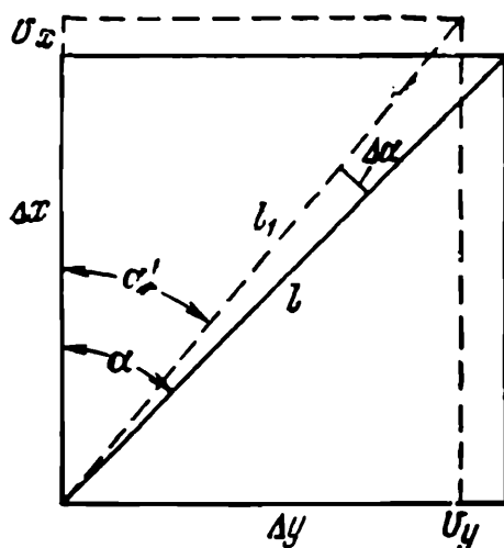
Рис. 122. Деформация бумаги
