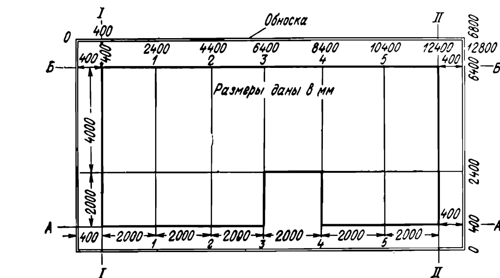
Рис. 175. Разбивочный чертеж обноска и внутренних осей фундамента
