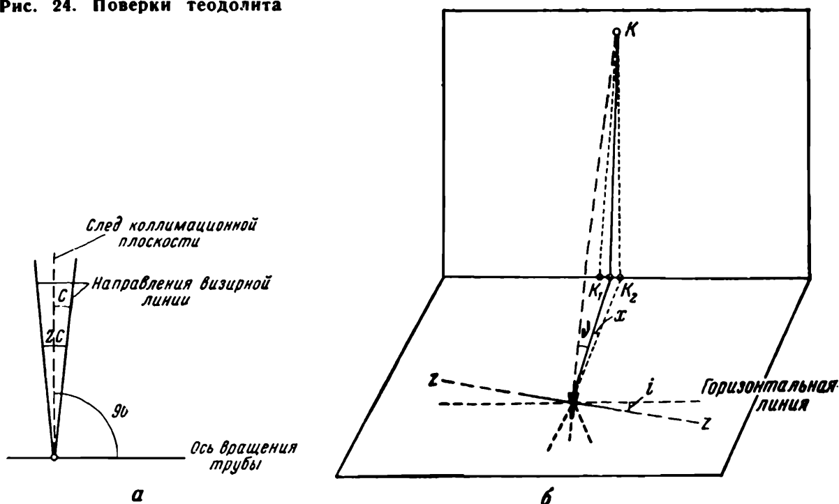
Рис. 24. Поверки теодолита
