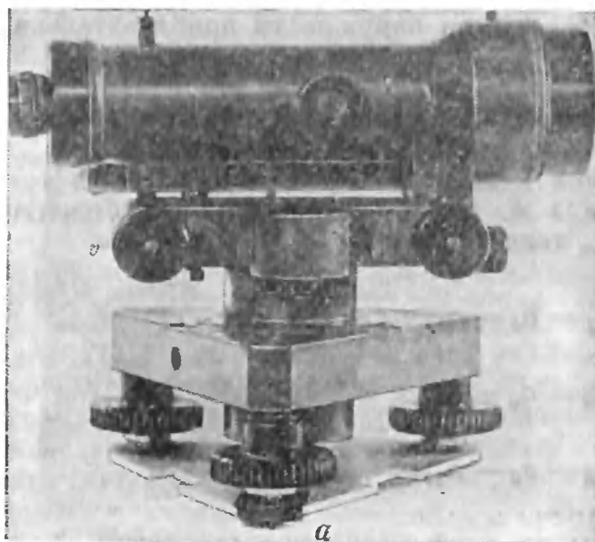
Рис. 73. Глухой нивелир НВ-1 (а) и поле зрения (б)
