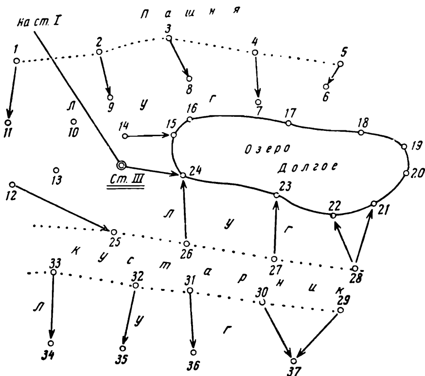
Рис. 100. Абрис на станции III
