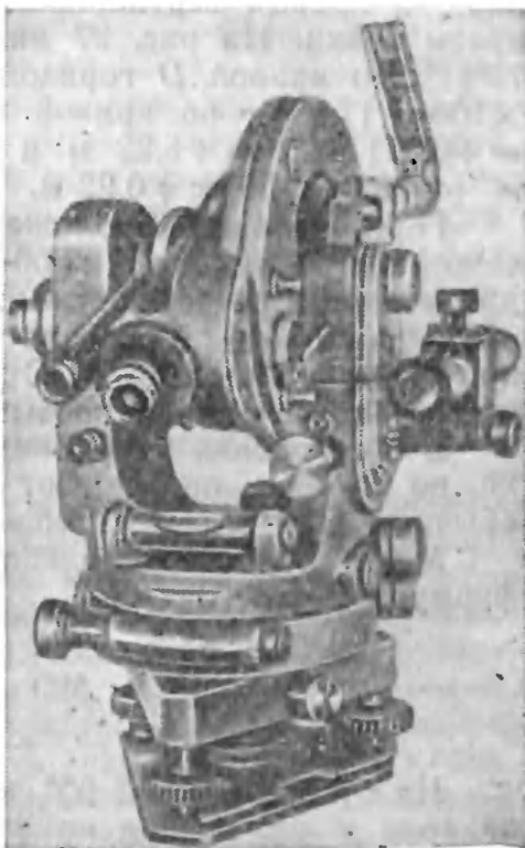
Рис. 96. Тахеометр-автомат ТА-2
