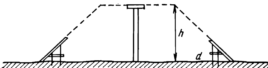
Рис. 162. Откосники и визирка для устройства насыпи
