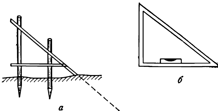
Рис. 161. Приспособления для разбивки откосов
