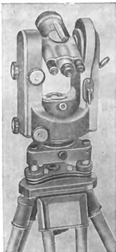
Рис. 19. Оптический теодолит ОТШ
