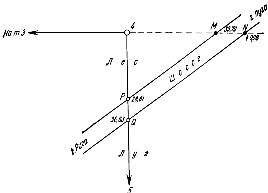
Рис. 55. Съёмка точек ситуации способом створов
