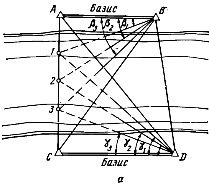
Рис. 189. Схема разбивки моста
