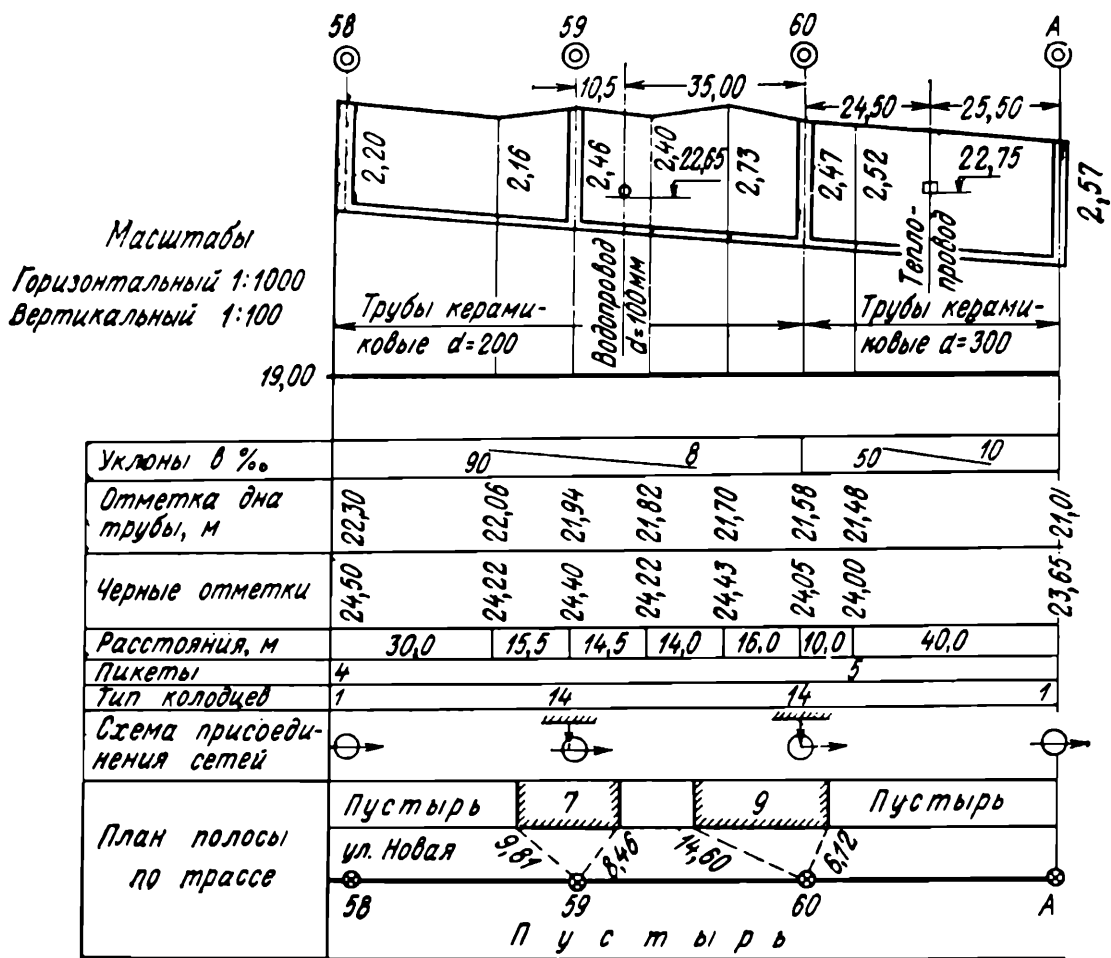
Рис. 84. Продольный профиль трассы канализации
