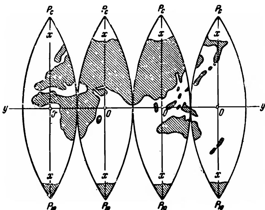
Рис. 35. Изображение координатных зон на плоскости
