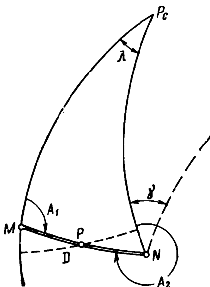
Рис. 27. Сближение меридианов
