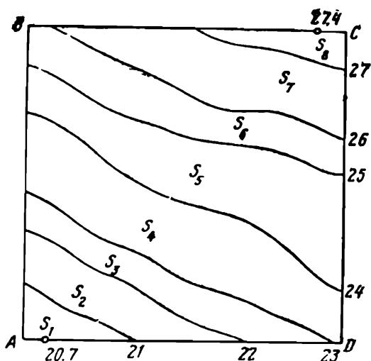
Рис. 132. Схема для вычисления общего объема тела по горизонталям
