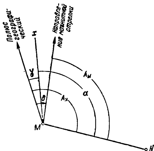
Рис. 31. Азимуты и дирекционный угол в восточной половине зоны при восточном склонении
