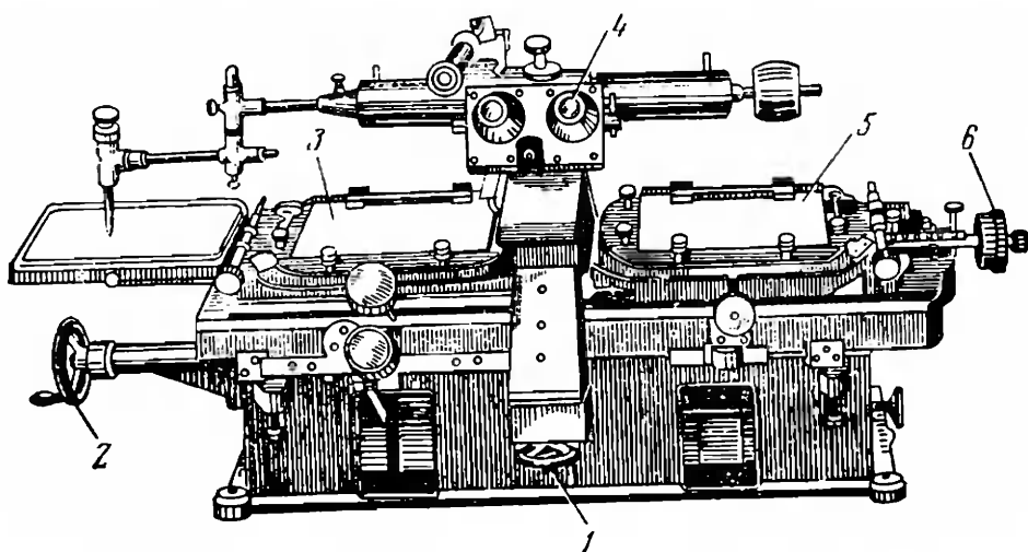
Рис. 108. Стереокомпаратор
